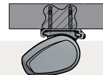
DECKENMONTAGE
