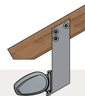
DACHSPARRENMONTAGE
